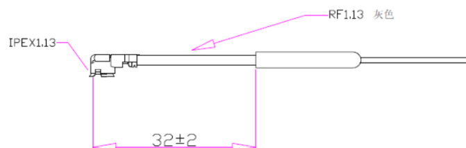
图 4 铜管天线尺寸
