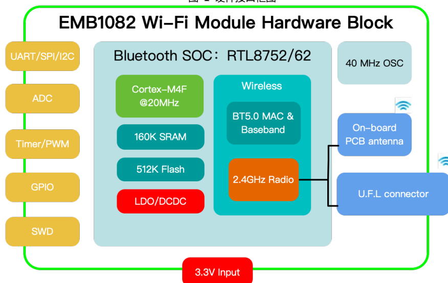
图 1 硬件接口框图
