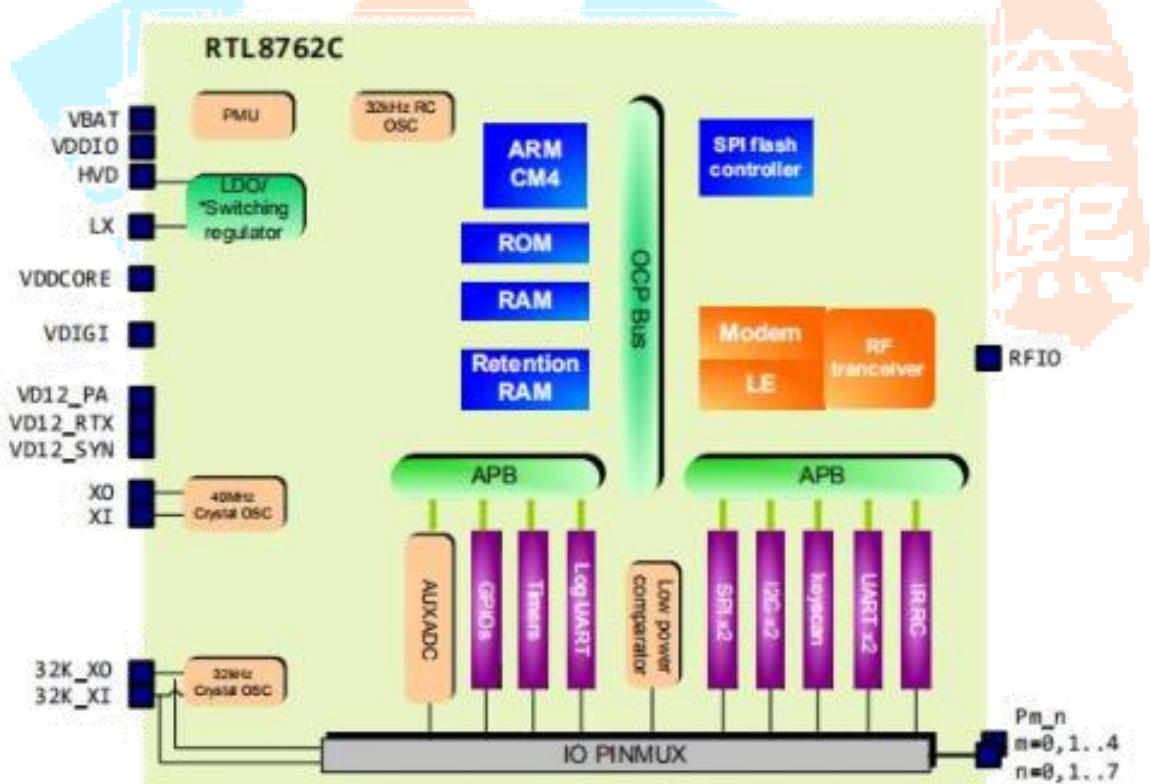
模组方框图
